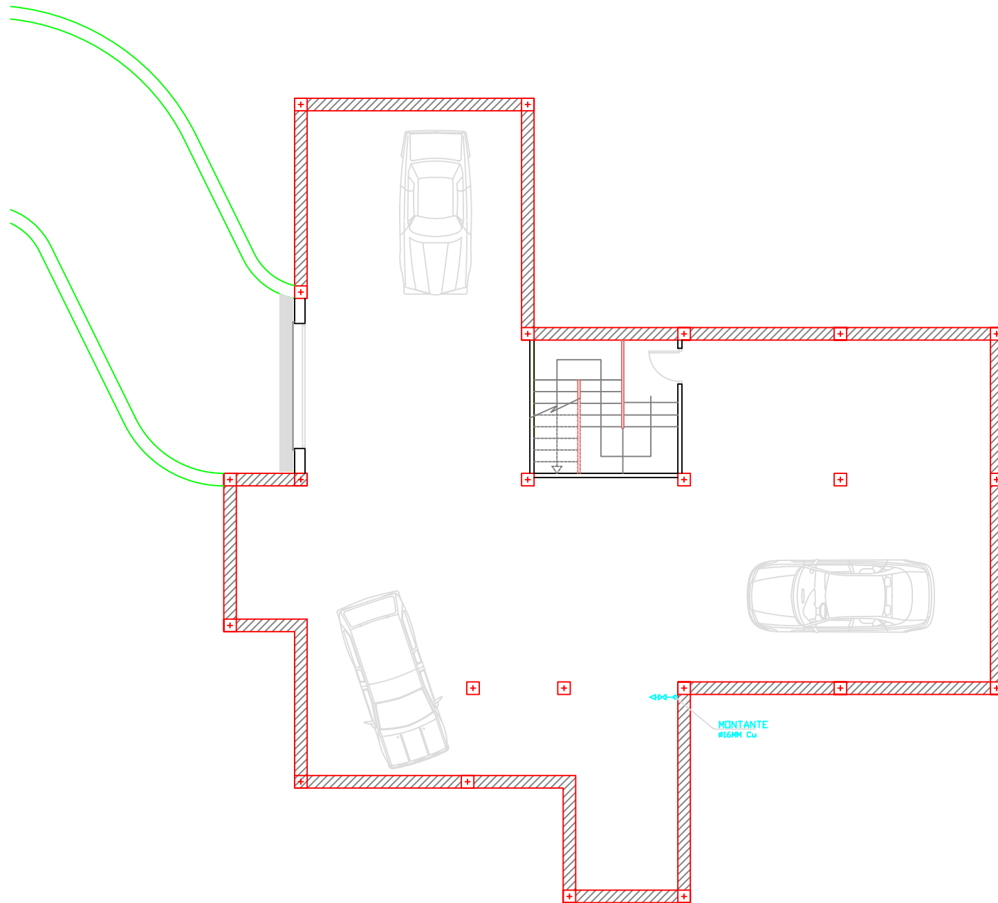
PLANTA SOTANO VILLA 1
